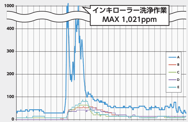
イ事業場のVOC濃度ピーク（前5分・後25分）
