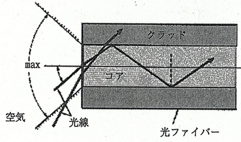
光ファイバーの構造
