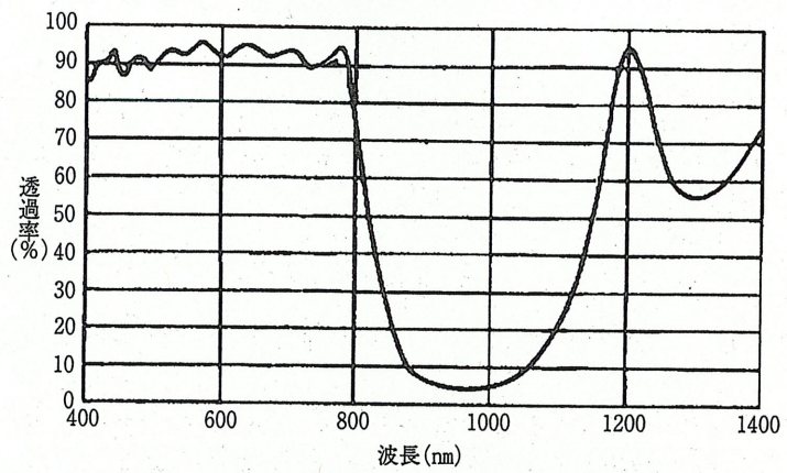
熱吸収ガラスの透過特性
