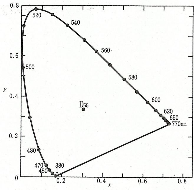
CIE XYZ 表色系
